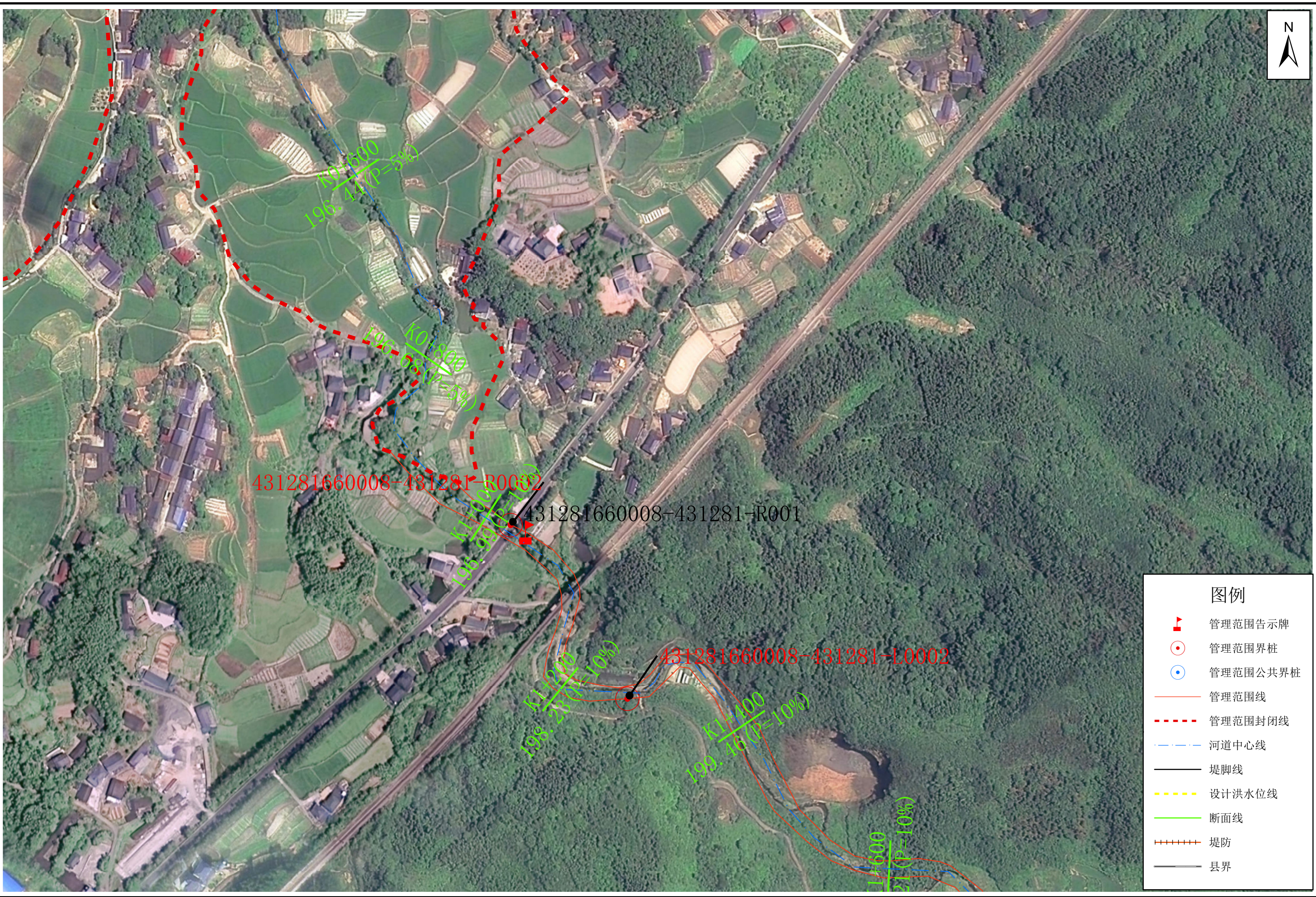
楠木堰溪怀化市洪江市河段管理范围划定图-2
